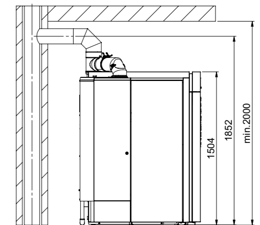
Seitenansicht – Abgassammler vertikal
