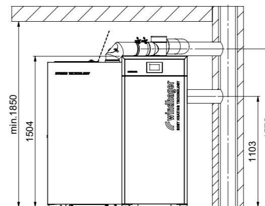
Frontansicht – getrennter Kaminanschluss
