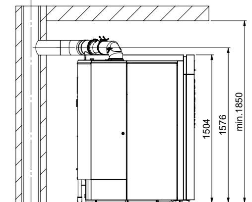
Seitenansicht – Abgassammler horizontal
