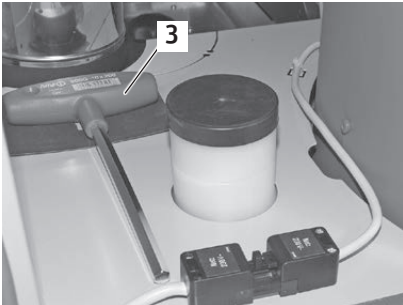
Fig. 54 Clé pour vis à six pans
