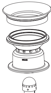
Fig. 100 Cône partie supérieure et partie inférieure, broche d'air primaire
