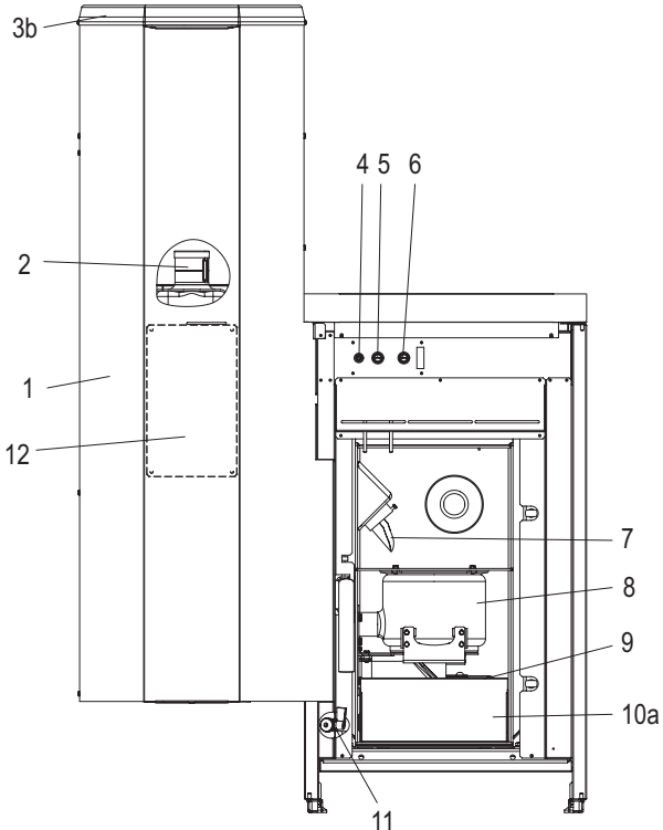
Fig. 10 Chaudière à pellets remplissage entièrement automatique sans porte de revêtement et sans porte de chambre à combustion
