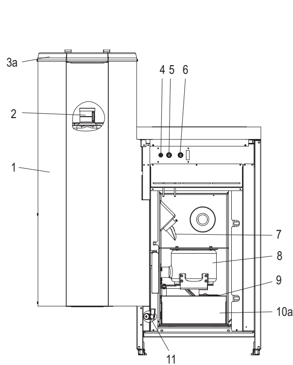
Fig. 9 Chaudière à pellets remplissage manuel sans porte de revêtement et sans porte de chambre à combustion
