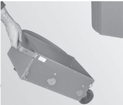
Fig. 85 Retirer le bac à cendres
