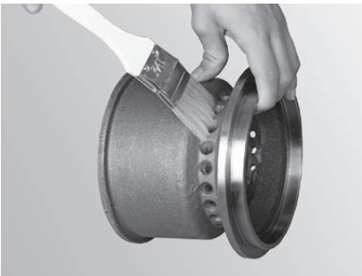
Fig. 93 Nettoyer le cône
