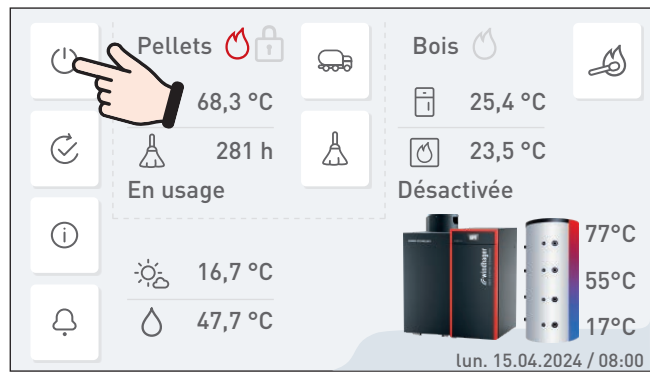
Fig. 47 Écran d'accueil chaudière à pellets
