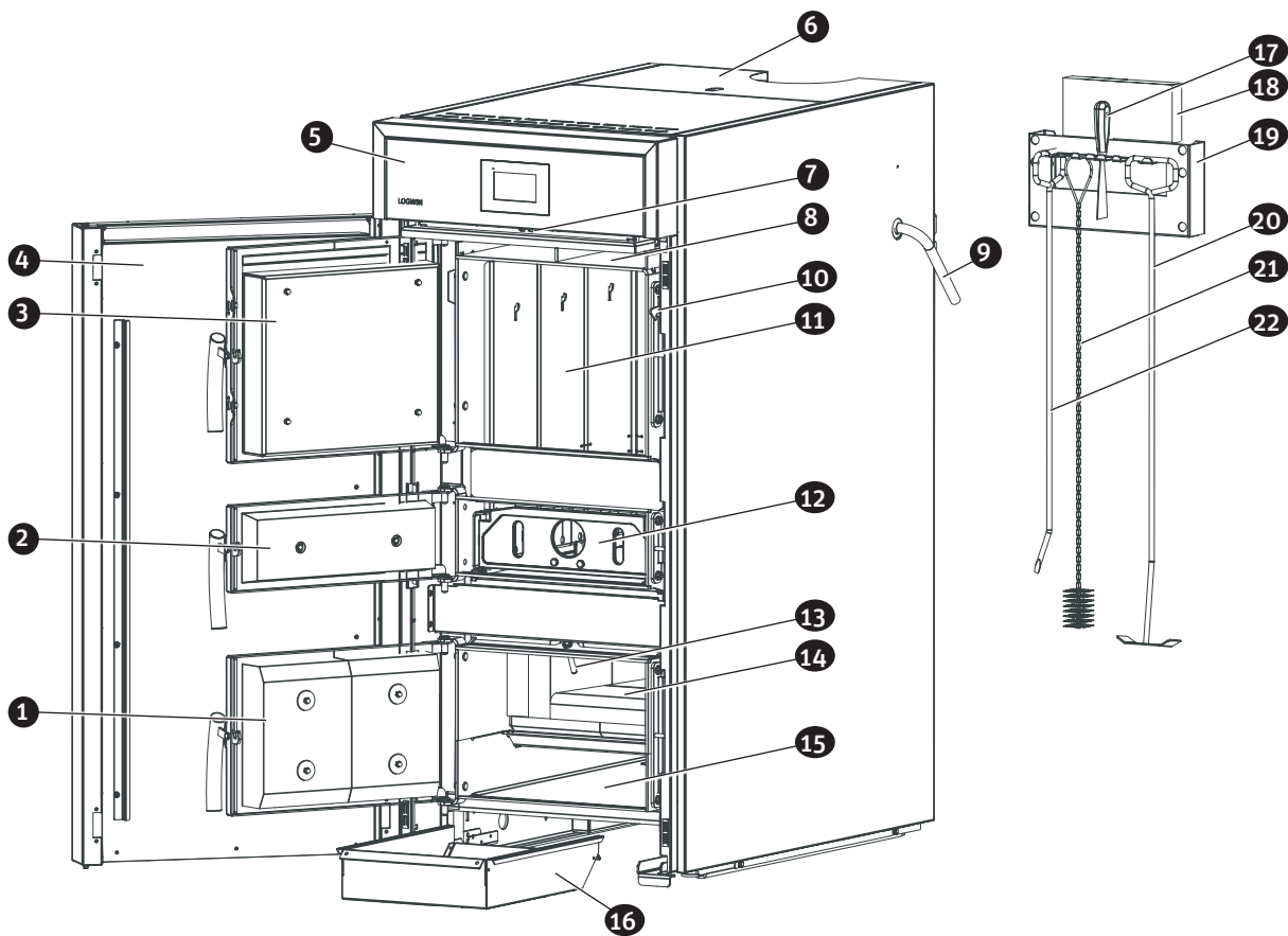
Fig. 16 Chaudière bois à gazéification LogWIN 2 EDEL
