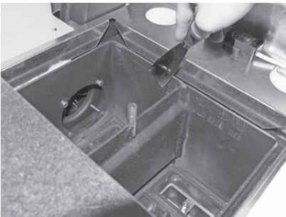
Fig. 109 Nettoyer les surfaces d'échange
