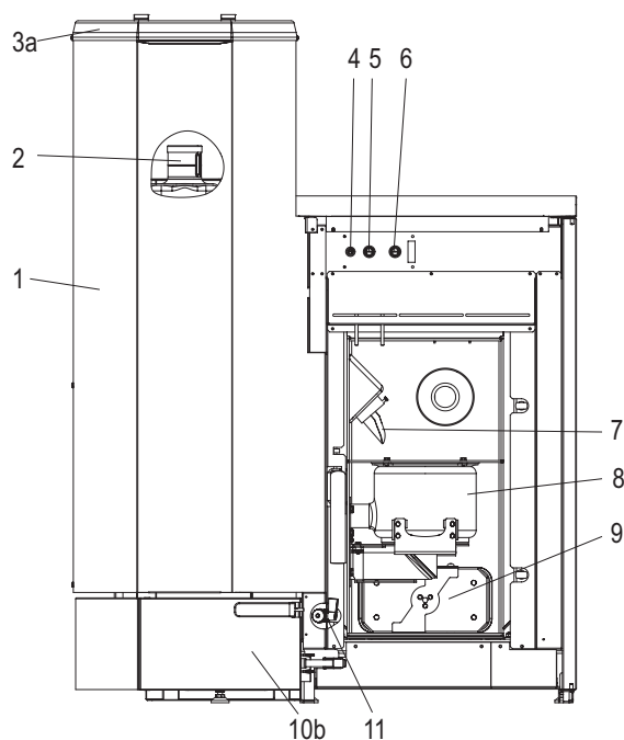
Fig. 11 Chaudière à pellets avec évacuation automatique des cendres dans un cendrier sans porte de revêtement et sans porte de chambre à combustion
