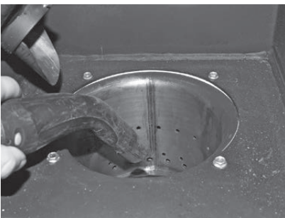
Fig. 95 Aspirer le creuset du brûleur
