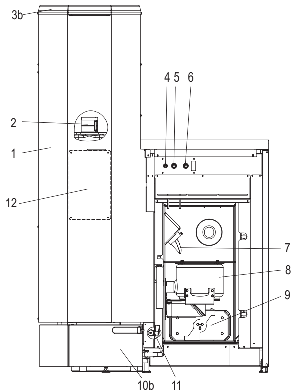
Fig. 12 Chaudière à pellets avec évacuation automatique des cendres dans un cendrier sans porte de revêtement et sans porte de chambre à combustion
