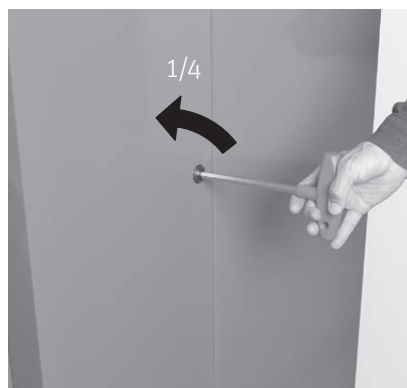
Fig. 7 Ouvrir la porte de revêtement à l'aide de la clé pour vis à six pans
