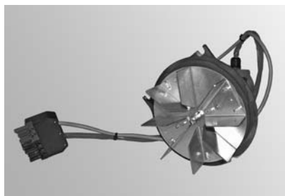
Abb. 151 Gebläserad reinigen
