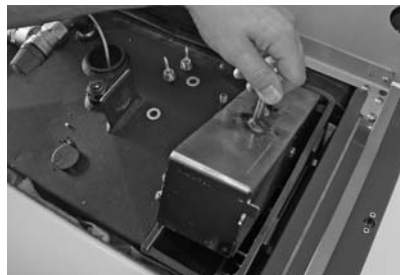
Abb. 144 Strahlschutzblech herausnehmen
