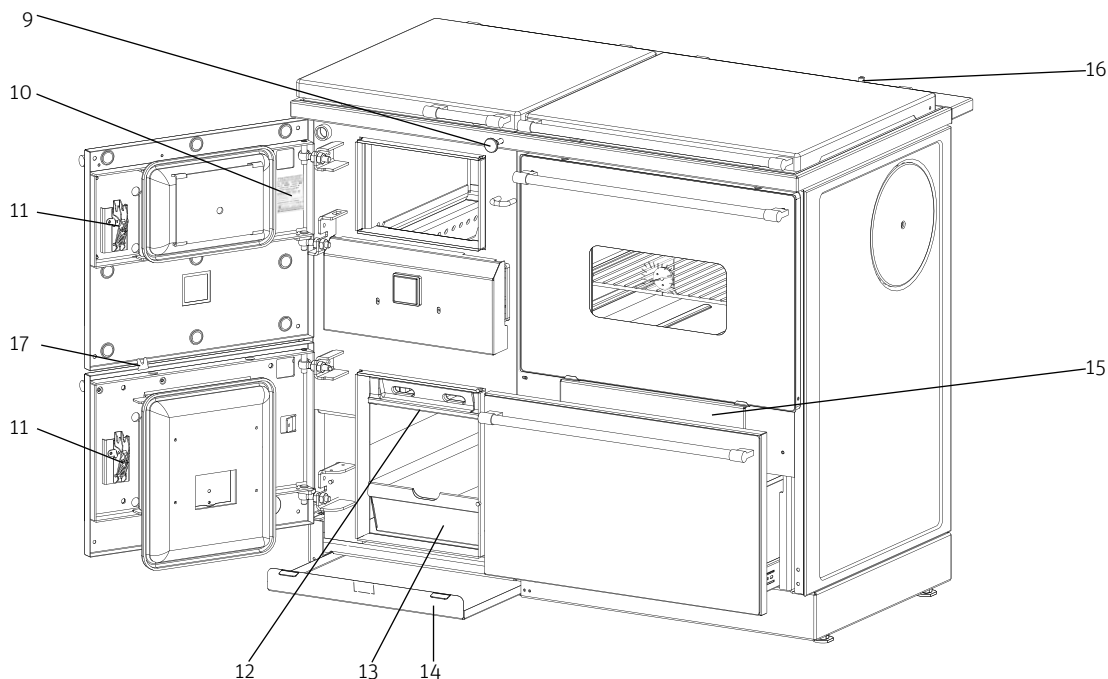
Fig.3 VestoWIN Premium; porte de chauffage et de cendrier ouverte
