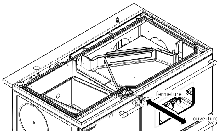
Fig.7 Ouverture/Fermeture du clapet de préchauffage – Vue sans table de cuisson en acier, ni plaque de cuisson en céramique
